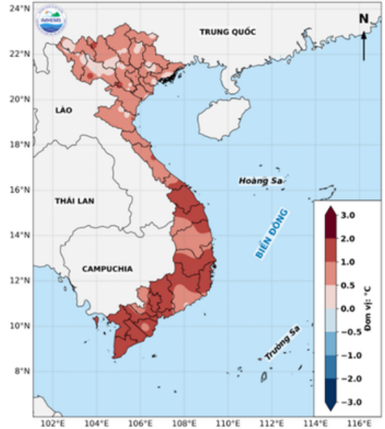
Hình 2. Phân bố chuẩn sai nhiệt độ trung bình mùa 3 tháng 6-8 năm 2026 (°C)
