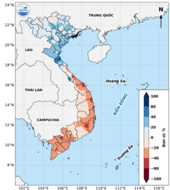
Hình 4. Phân bố chuẩn sai lượng mưa mùa 3 tháng 6-8 năm 2026 (%)
